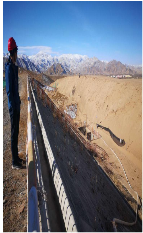
坝脚排水沟
